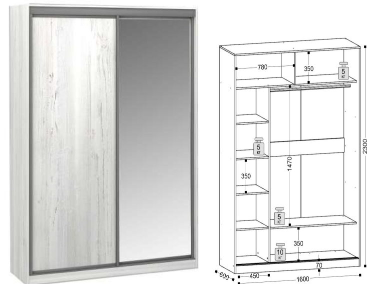
6.16.1 Шкаф-купе без зеркала ш-1600, г-600, в-2300
