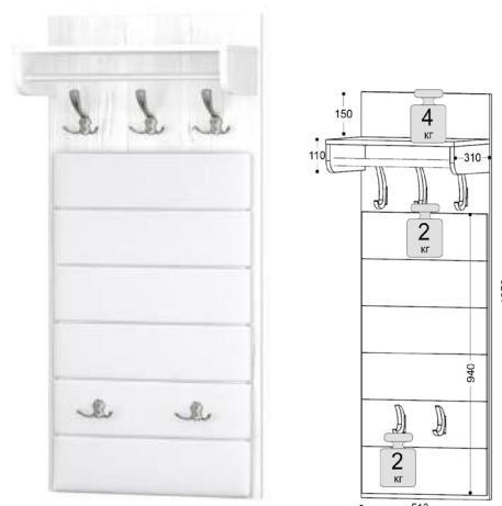
6.1 Вешалка настенная ш-510, г-310, в-1350
