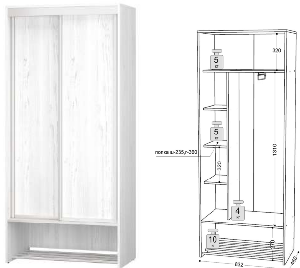
10.1 Шкаф-купе без зеркала ш-832, г-460, в-2000
