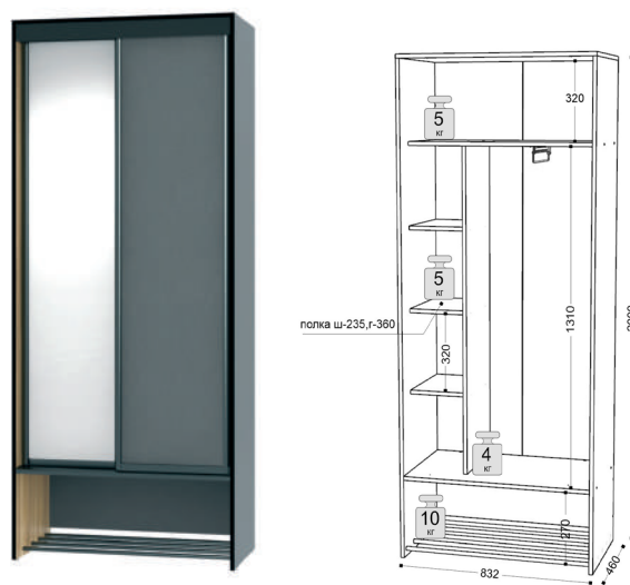
10 Шкаф-купе с зеркалом 10.1 Шкаф-купе без зеркала ш-832, г-460, в-2000
