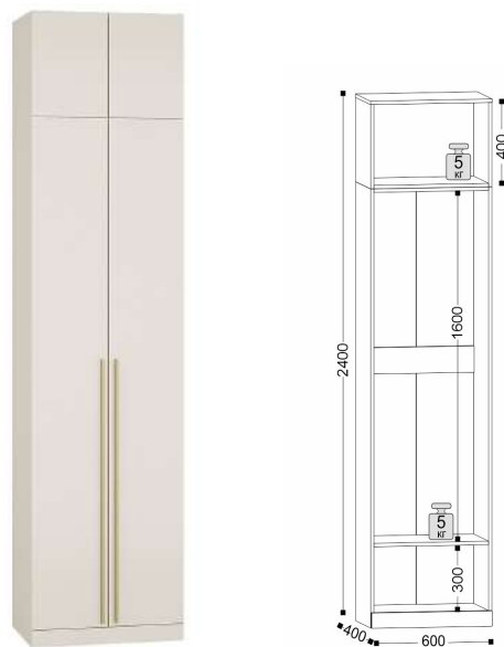
20 Шкаф 2-х створчатый ш-600, г-400, в-2400
