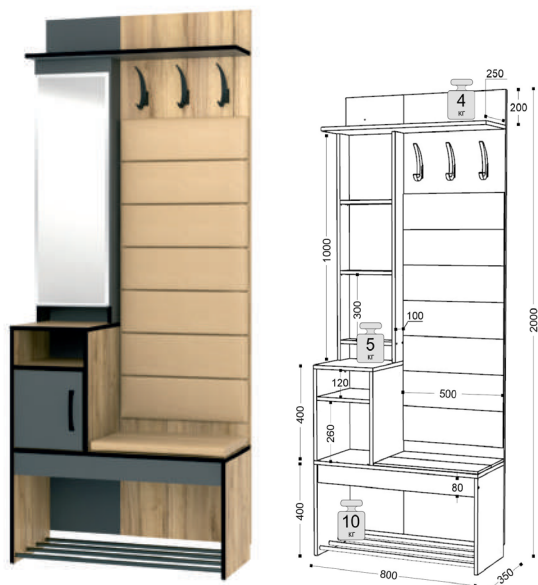
1 Прихожая ш-800, г-350, в-2000
