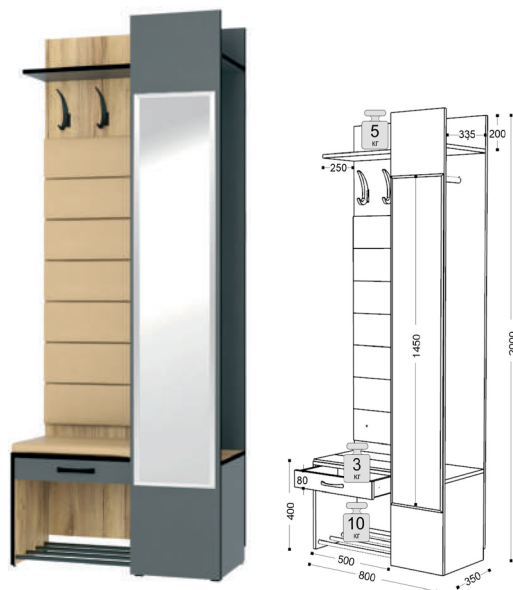
2 Прихожая ш-800, г-350, в-2000
