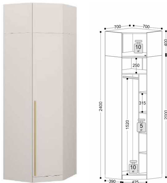
26 Шкаф угловой ш-700, г-700, в-2400
