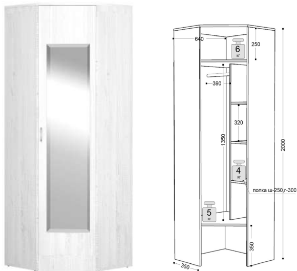
9.2 Шкаф угловой с зеркалом ш-660, г-660/350, в-2000
