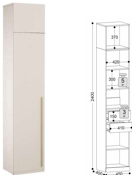
6 Пенал ш-450, г-400, в-2400
