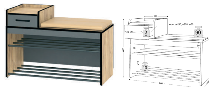
5 Тумба ш-800, г-350, в-600
