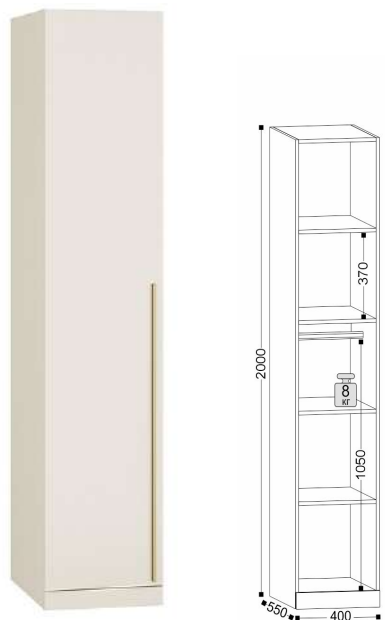
62 Пенал ш-400, г-550, в-2000
