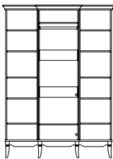
шкаф для платья и белья ГМ 6553-10, 2192 x 1614 x 628
