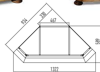
шкаф (угловой) ГМ 5613Е, 2114 x 1322 x 589
